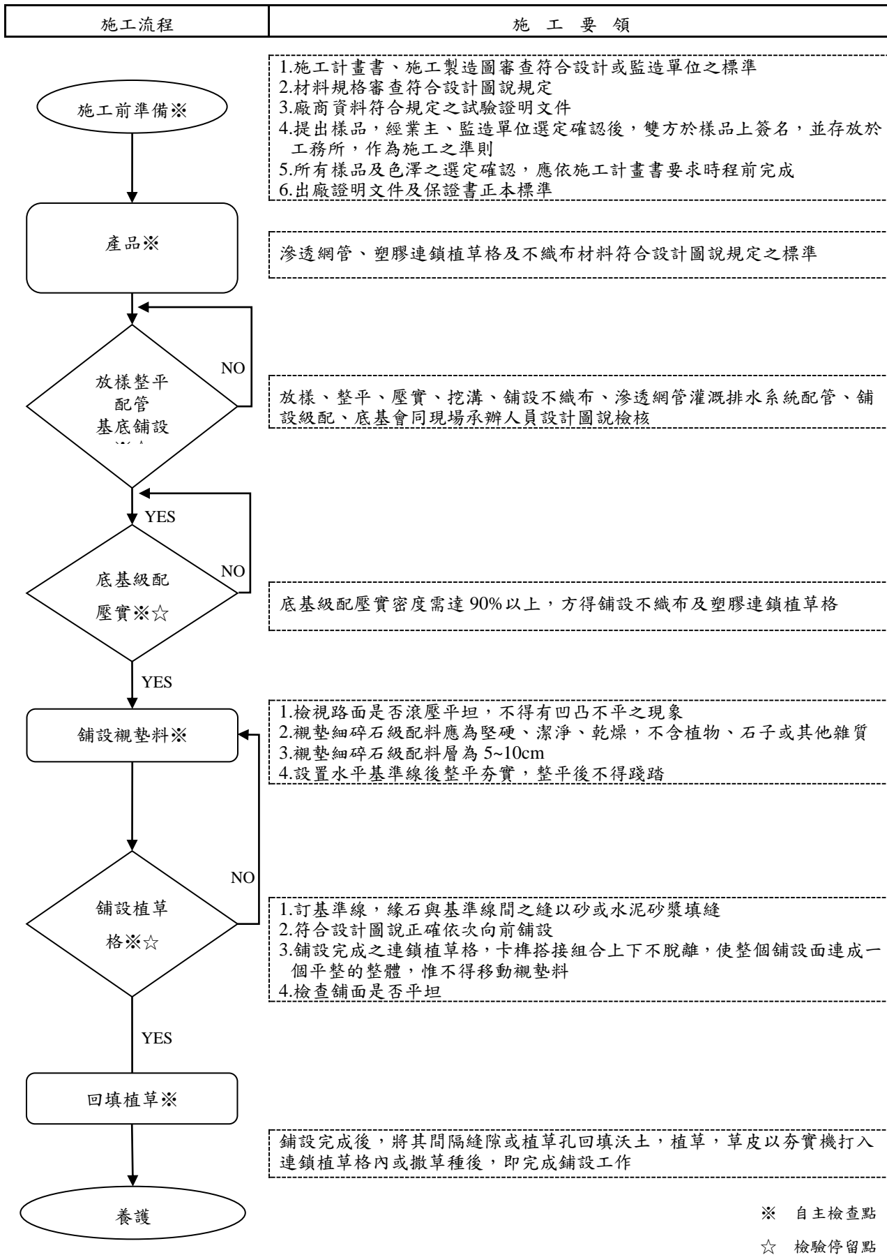
圖 11-1 貳、滲透網管地下灌溉排水綠化系統停車場工程施工要領作業流程圖
