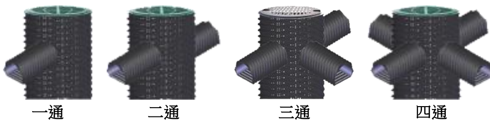
網管陰井管徑 + 滲透網管配置表
